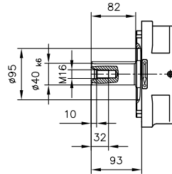
键轴 标记 K ( \varnothing 40 - A12x8x80 DIN 6885)
