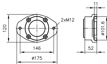
标记 C424、C426 ( SAE-B 2 孔和 SAE-B 4 孔 )
