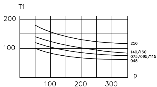
p 压力 (bar) ; 控制时间 T_1 (ms)
