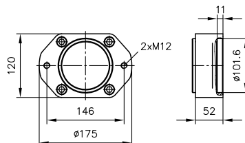
标记 C474、C476 ( SAE-B 2 孔和 SAE-B 4 孔 )
