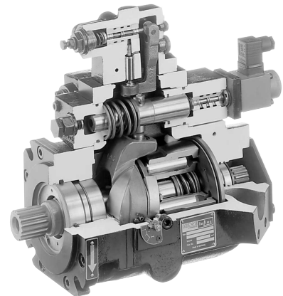
V30D 型轴向柱塞变量泵
