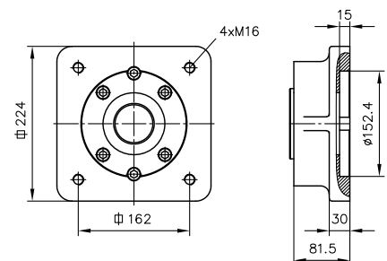
标记 C480 ( SAE-D 4 孔 )
