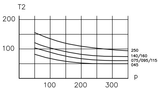
p 压力 (bar) ; 控制时间 T_2 (ms)
