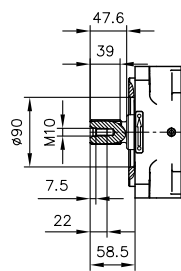
花键轴 标记 S (SAE-C J744 14T 12/24 DP)
