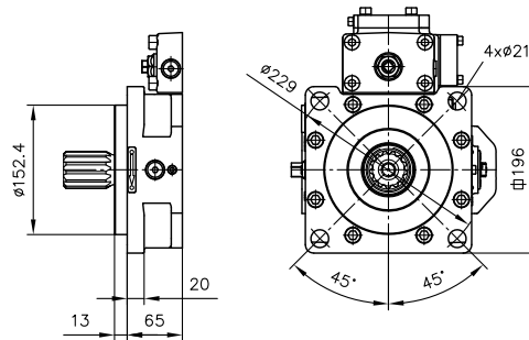
标记 F (SAE-D 4 孔 J 744) (152-4 DIN ISO 3019-1)
