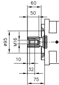
花键轴 标记 S (SAE-D J744 13T 8/16 DP)
