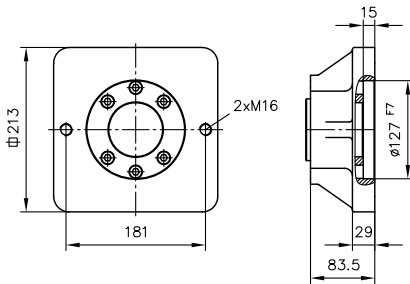
标记 C427、C429 ( SAE-C 4 孔和 SAE-C 2 孔 )
