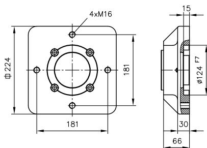
标记 C477、C479 ( SAE-C 4 孔和 SAE-C 2 孔 )
