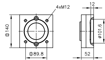
标记 C425 ( SAE-B 4 孔 )
