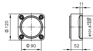
标记 C475 ( SAE-B 4 孔 )
