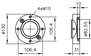
标记 C421、C422、C423 ( SAE-A 2 孔 )
