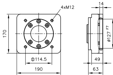
标记 C428 ( SAE-D 4 孔 )
