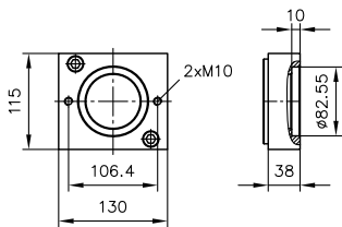
标记 C471、C472、C473 ( SAE-A 2 孔 )
