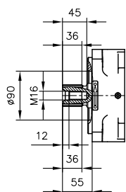
花键轴 标记 D (W40x2x18x9g DIN 5480)
