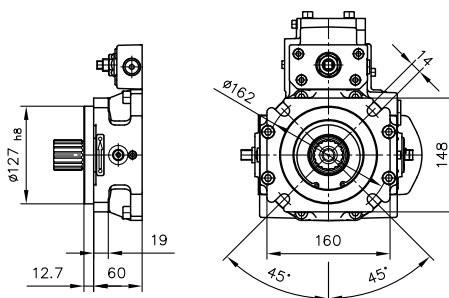
标记 F (SAE-C 4 孔 J744) (152-4 DIN ISO 3019-1)
