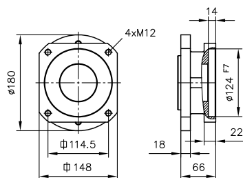
标记 C478 ( SAE-D 4 孔 )
