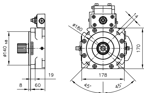
标记 G (140 B4 HW DIN ISO 3019-2)
